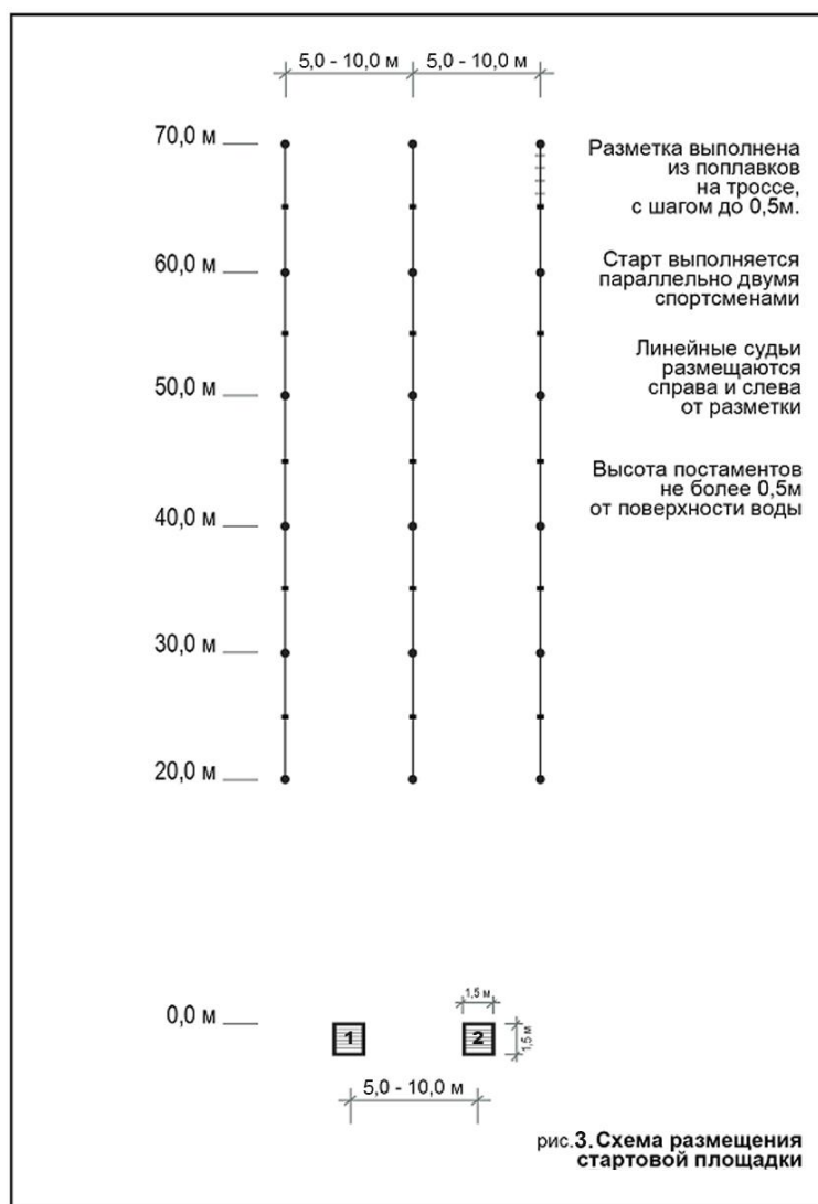
Рисунок 9. Схема установки стартовой площадки для дисциплины «Кастинг нахлыстовый – дальность-лосось».
