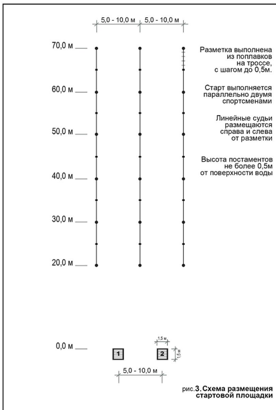
Рисунок 7. Схема установки стартовой площадки для дисциплины «Кастинг нахлыстовый – дальность-морская форель».
